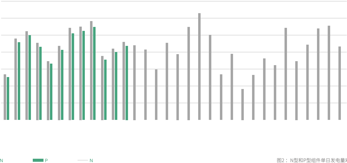
图2：N型和P型组件单日发电量对比
